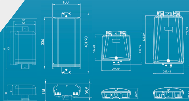
Tampa deslizante
